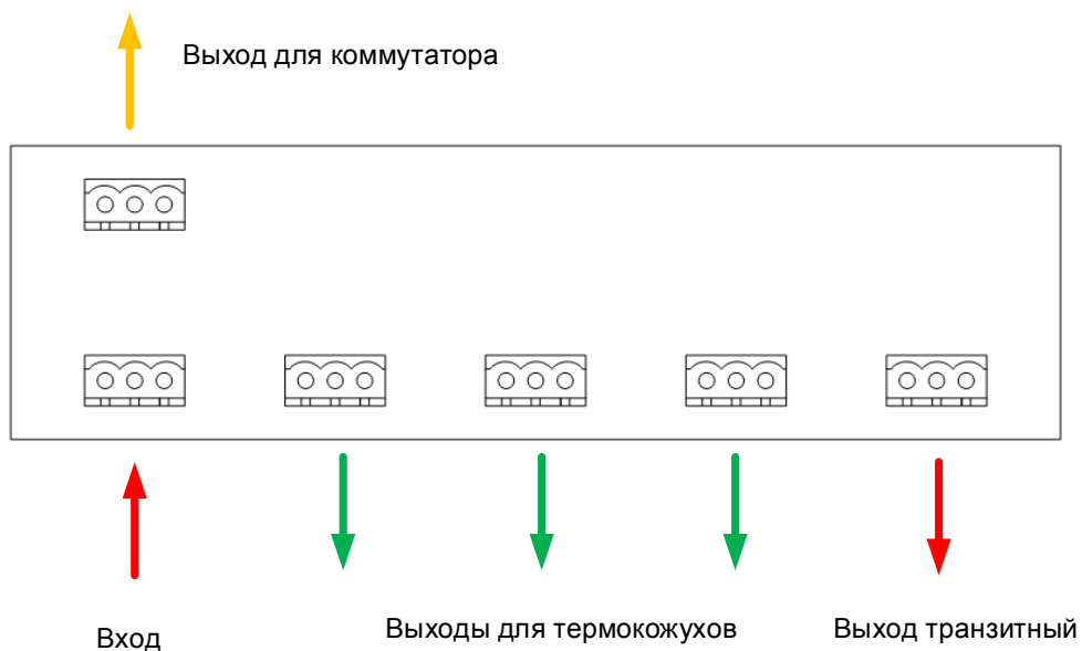
Рис. 2.5-1. Назначение разъемов
