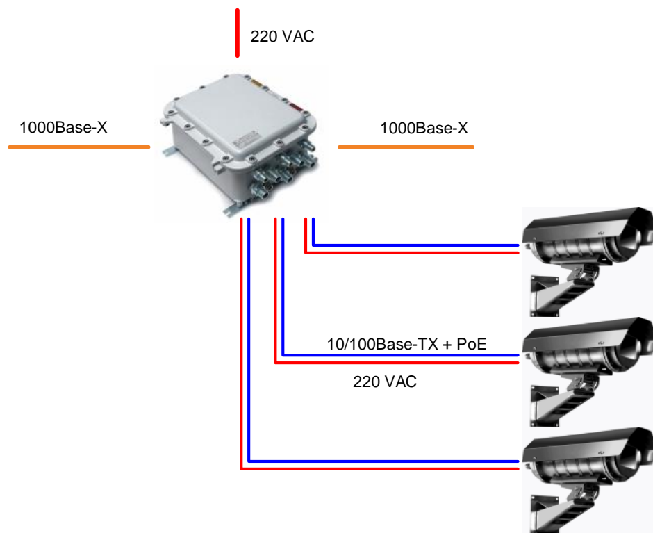
Рис. 1. Схема подключения PSW-2G4F-Ex
