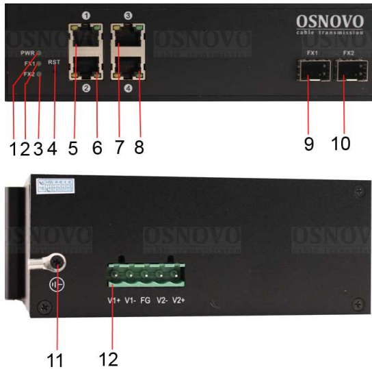
Рис. 3 Разъемы и индикаторы коммутатора SW-8042/IC
